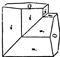
Calcite.
